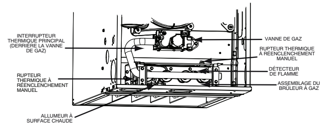
Fig. 27 – Ensemble de brûleurs à gaz (tirage descendant)
