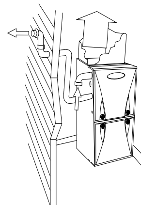
Fig. 3 – Tuyau d'air de combustion intérieur
