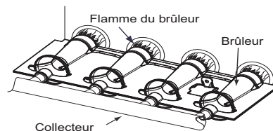
Fig. 5 – Réglage de la flamme des brûleurs DÉMARRAGE DE LA CHAUDIÈRE
