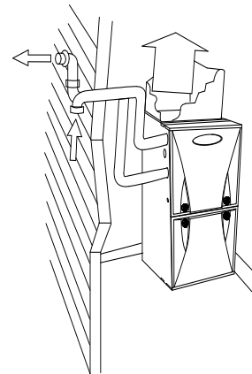
Fig. 2 – Tuyaux d'évent extérieurs
