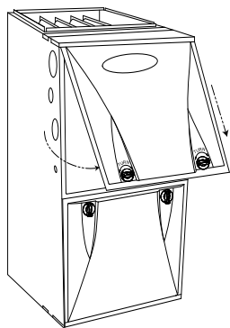
Fig. 10 – Retrait de la porte principale de la chaudière (configuration à tirage ascendant)
