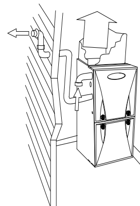
Fig. 3 – Tuyau d'air de combustion intérieur
