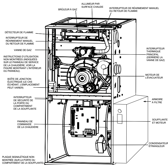
Fig. 1 – COMPOSANTS DE LA CHAUDIÈRE
