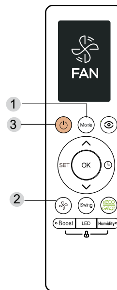
Figure 8 – Mode FAN (VENTILATION)
